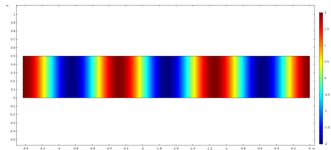
Abbildung 4: Simuliertes Schalldruckfeld in einem 3,4 m langen Impedanzrohr bei einer Frequenz von 300 Hz und einer schallharten Randbedingung am Ende des Rohrs.
