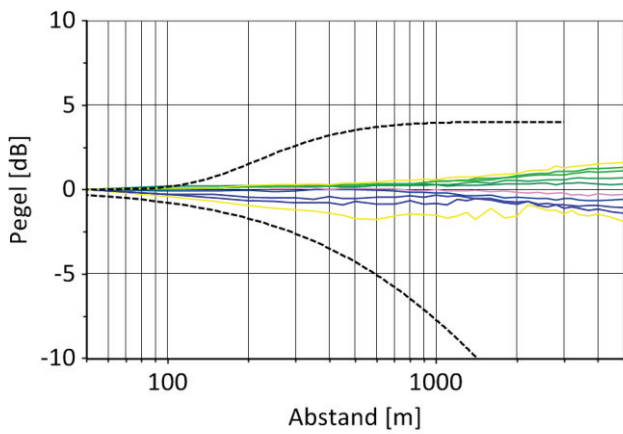
Abbildung 1 Abstandsabhängigkeit der Perzentile Szenario: Industriergeräusch, freie Schallausbreitung von oben nach unten CRM, HAR, ISO, ISA
