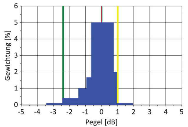
Abbildung 2 Rekonstruierte Potentialverteilung in 800 m Abstand Szenario: Industriergeräusch, freie Schallausbreitung von oben nach unten CRM, HAR, ISO, ISA
