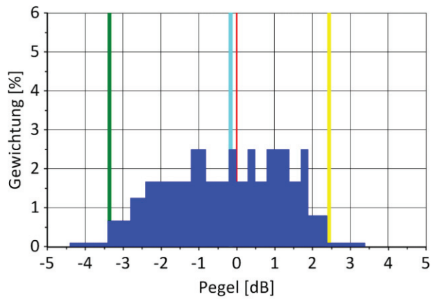
Abbildung 4 Rekonstruierte Potentialverteilung in 800 m Abstand Szenario: Gewehrschuss im Schießstand, geschirmt von oben nach unten CRM, HAR, ISO, ISA
