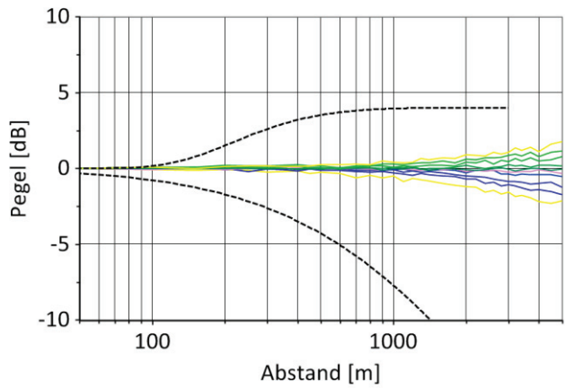
Abbildung 3 Abstandsabhängigkeit der Perzentile Szenario: Gewehrschuss im Schießstand, geschirmt von oben nach unten CRM, HAR, ISO, ISA
