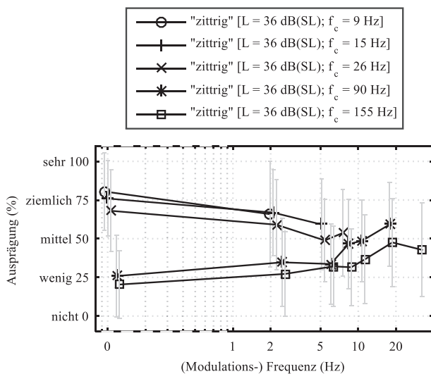
Abbildung 8: Ausprägung des Attributs „zittrig“ für sinusoidale Signale im Vergleich zu AM-sinusoidalen Signalen in Abhängigkeit der Modulationsfrequenz
